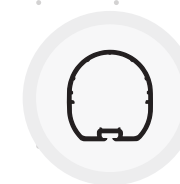
Torrahmenprofil P0077 120 x 100 mm
